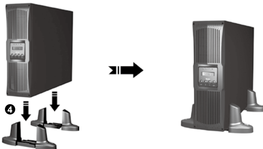
Рис. 3ф. Установка ИБП в опоры для вертикальной установки
