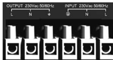
Рис. 3h. 10 кВА
