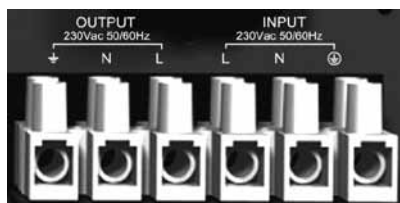
Рис. 3г. 5 кВА/6 кВА
